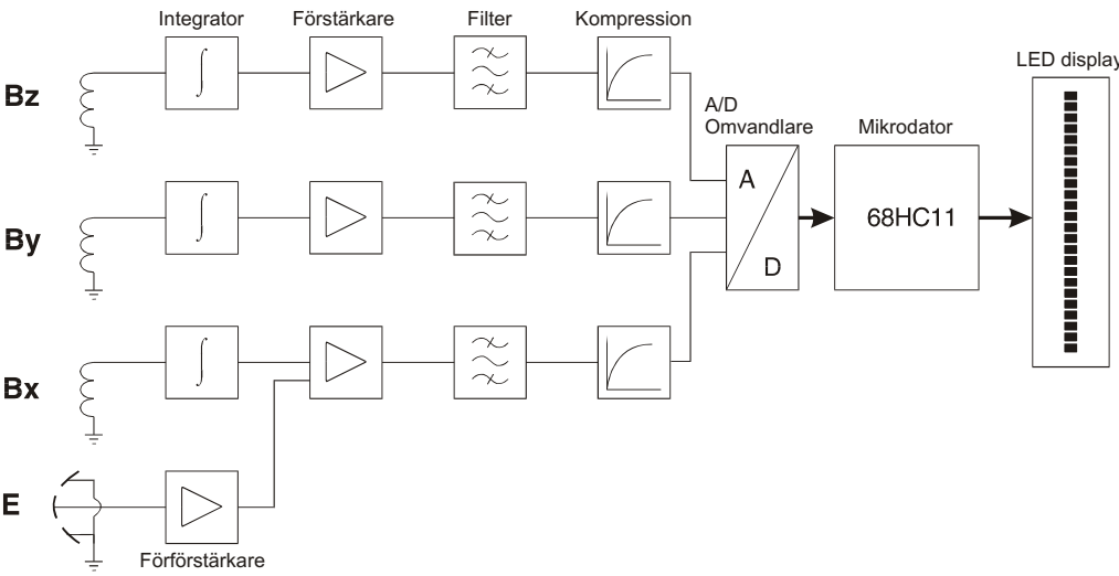
Fig. 4.1 FD1 blockdiagram
