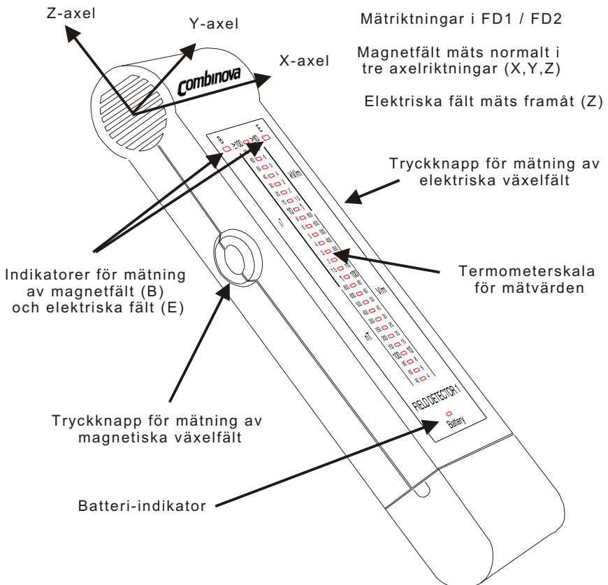
Figur 3.1 FD1 / FD2 - Mätriktningar, tryckknappar och indikatorer.
